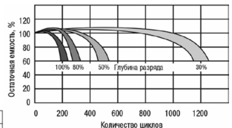
Рис. 11б. Зависимость циклического ресурса от глубины разряда для серии ВР
