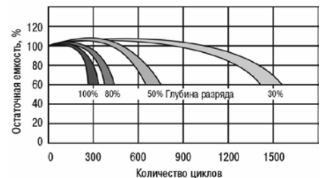
Рис. 11г. Зависимость циклического ресурса от глубины разряда для серий UPS, FTB, FTH
