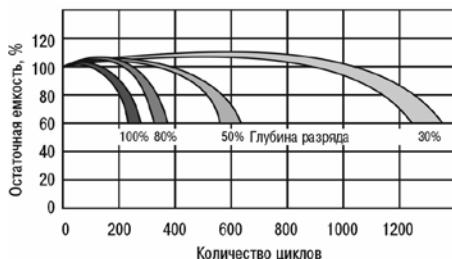
Рис. 11в. Зависимость циклического ресурса от глубины разряда для серий BPS и HRL
