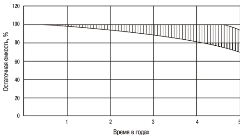
Рис. 12. Срок службы аккумулятора, работающего в режиме постоянного подзаряда
