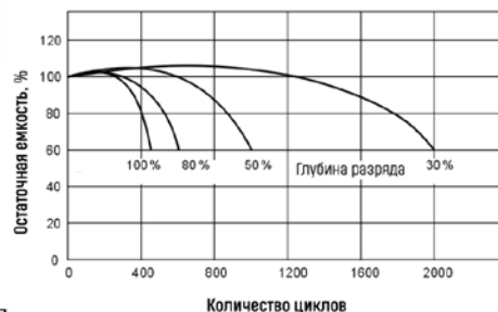
Рис. 11д. Зависимость циклического ресурса от глубины разряда для серии MSU
